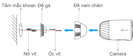
Hình 1 Gắn bằng đế nam châm
