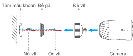
Hình 2 Gắn bằng đế vít
